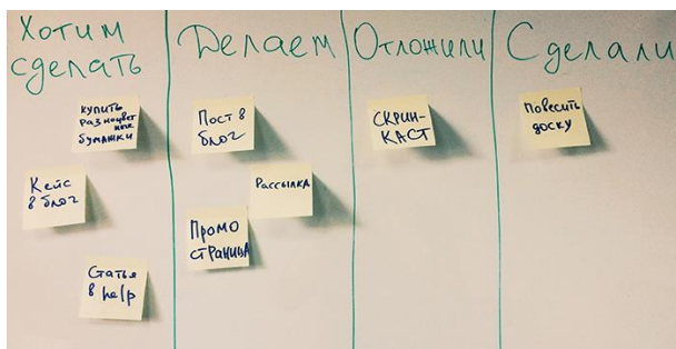
Рисунок 1 – Пример Канбан-доски.
