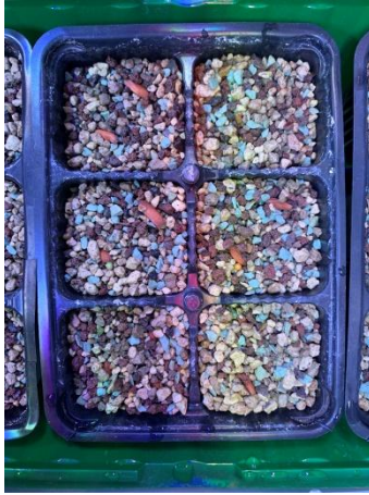
Рисунок 2 – Проросшие семена
