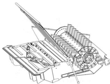
Рисунок 1 – Устройство измельчителя КЗС-1218
