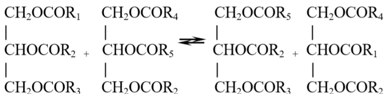
Рисунок 4 – Схема переэтерификации жиров
