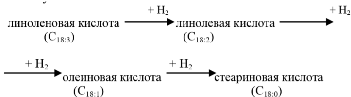
Рисунок 1 – Схема химических превращений при каталитическом гидрировании жирных кислот
