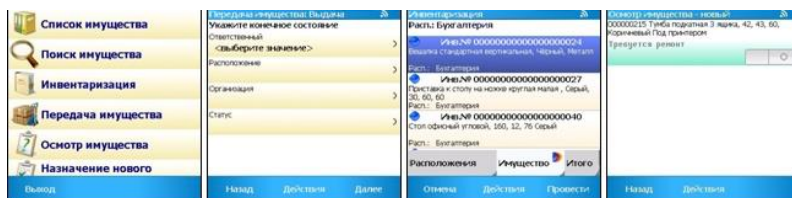
Рисунок 4 – Мобильный клиент
